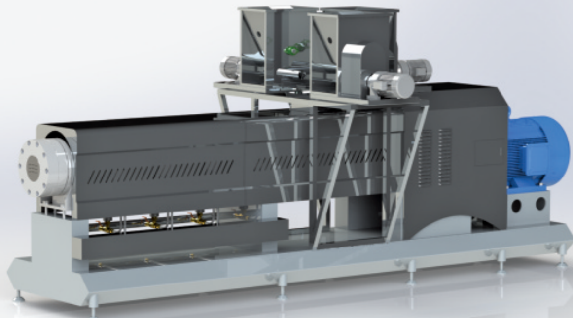
TPS100-T 三色挤出机 TPS100-T Tri-Color Extruder
