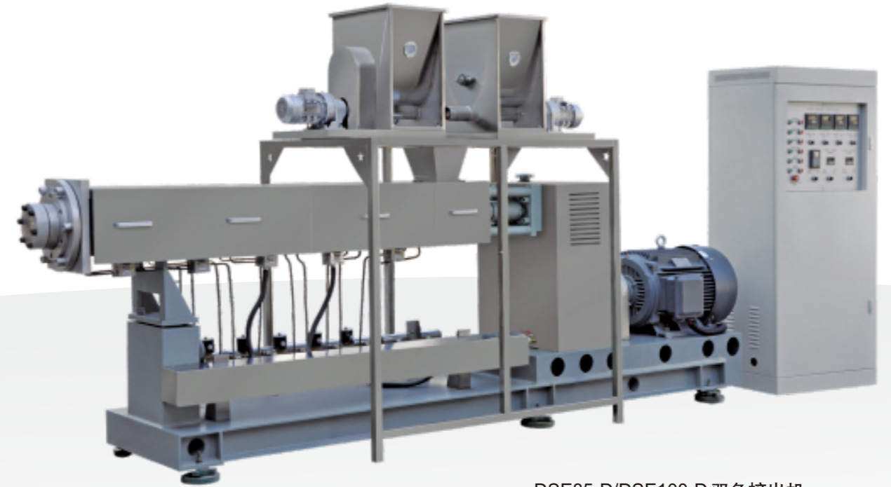
DSE85-D/DSE100-D 双色挤出机 DSE85-D/DSE100-D Double Color Extruder
